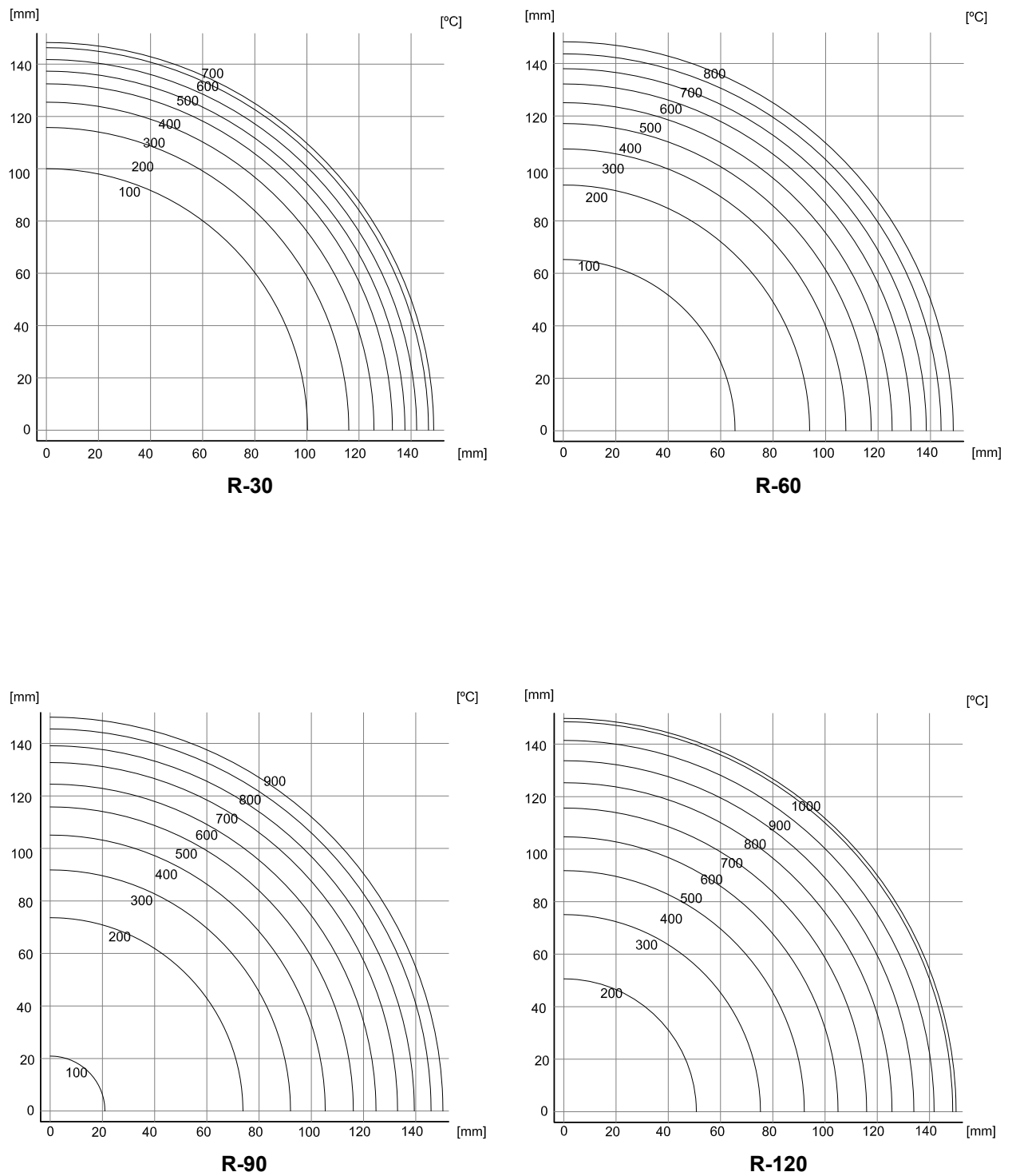
Figura C.7. Isotermas de un cuarto de sección circular de 300 mm de diámetro expuesta perimétralmente
